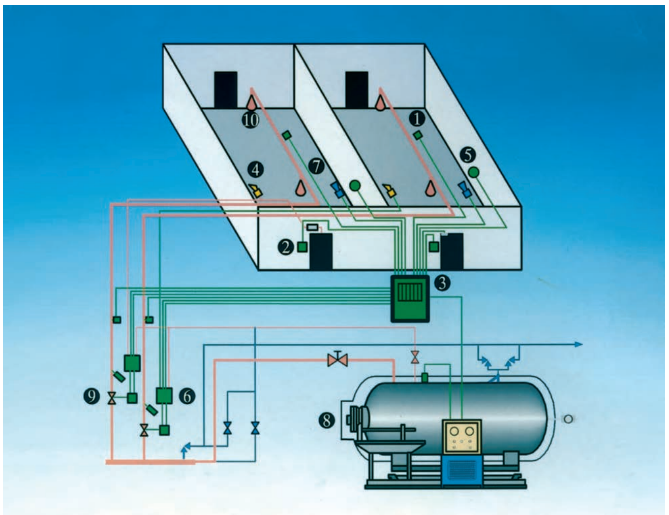
Systemdarstellung der CO 2 -Niederdruckanlage
