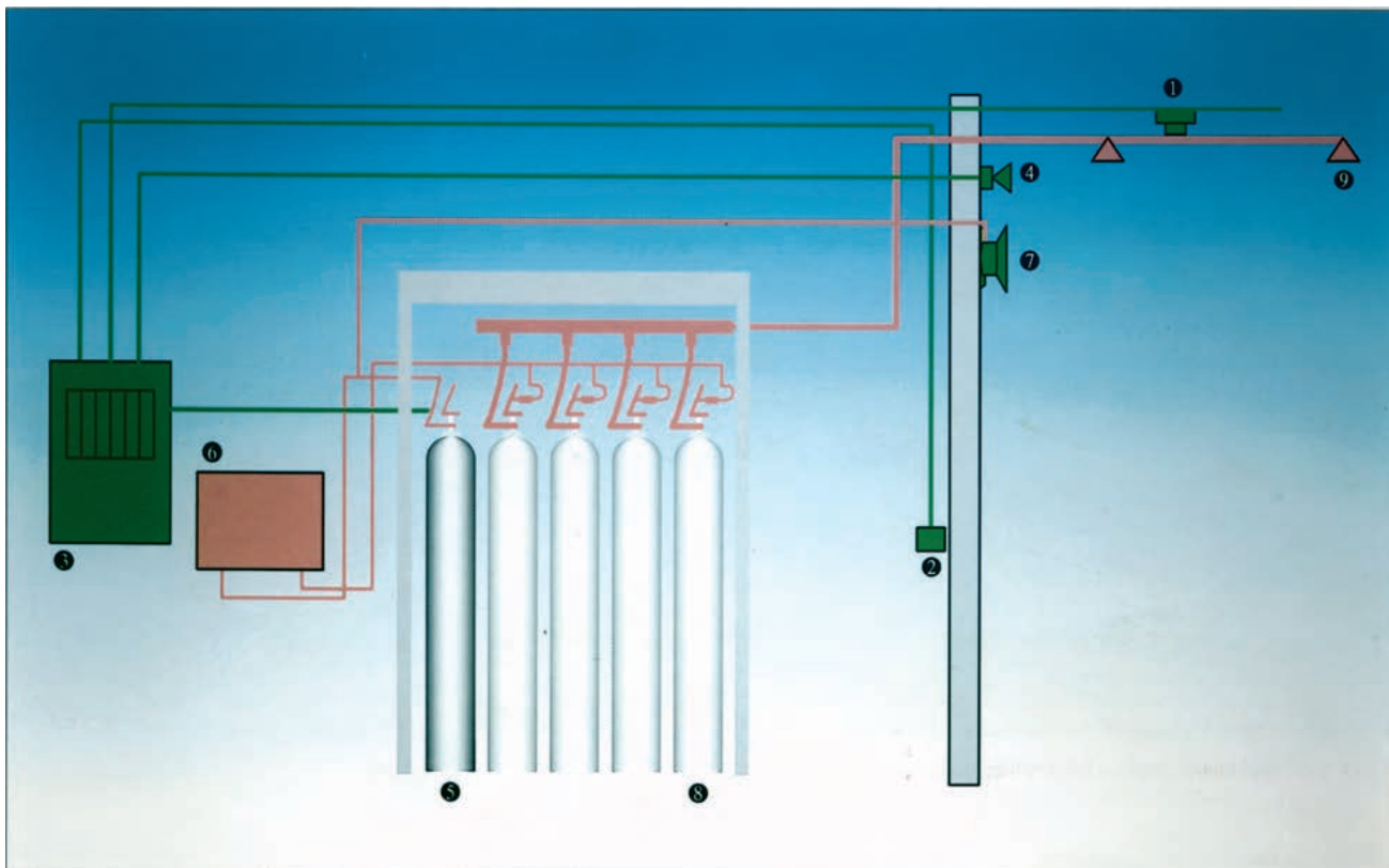
Systemdarstellung der CO 2 -Hochdruckanlage
